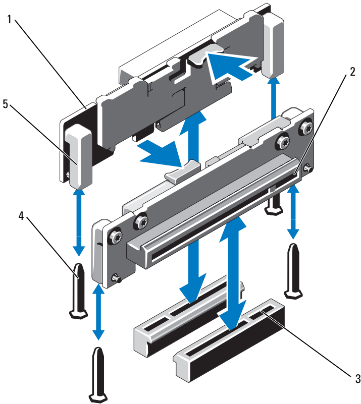
Figure 3-11. Installation et retrait d'une carte de montage
