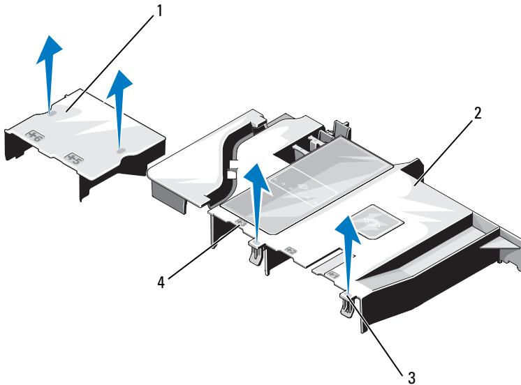
Figure 3-13. Installation et retrait du carénage de refroidissement
