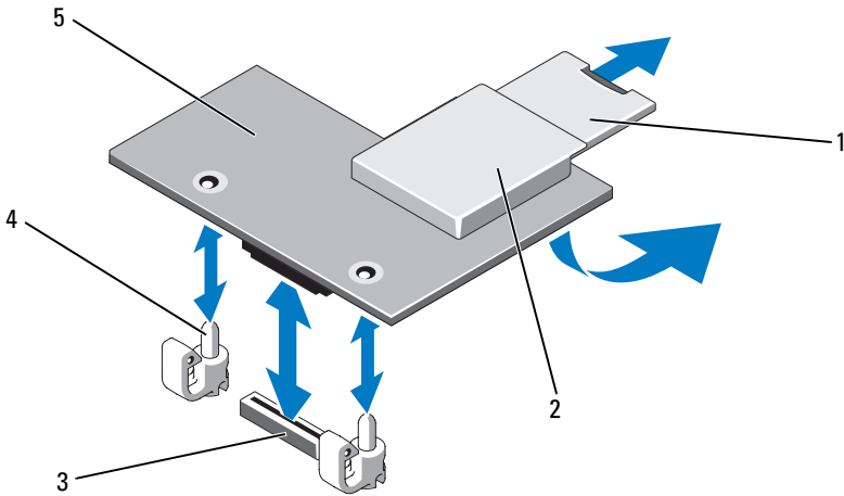
Figure 3-18. Installation et retrait d'une carte iDRAC6 Enterprise
