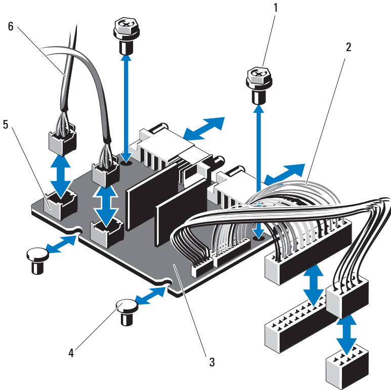
Figure 3-26. Carte de distribution de l'alimentation
