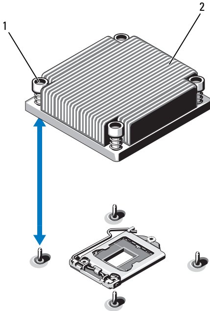
Figure 3-19. Installation et retrait du dissipateur de chaleur
