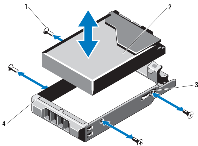
Figure 3-9. Retrait et installation d’un disque dur dans un support de lecteur
