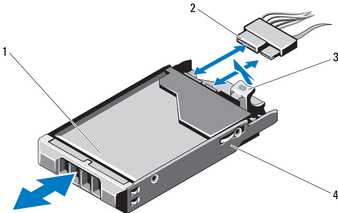
Figure 3-8. Retrait et installation d'un disque dur connecté par câble
